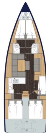
5-Kabinen-Layout
